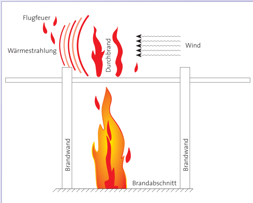
Abb. 3: Mechanismen der Brandweiterleitung auf der Dachoberseite: Das Nachbardach kann, ausgehend vom Durchbrand, durch Windeinwirkungen, Flugfeuer und durch Strahlung beeinträchtigt werden. Brandwände sollen dies verhindern.
