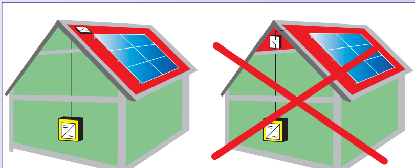
Abb. 6: Bei Isolationsschäden ungeschützter (roter) und geschützter (grüner) Bereich einer PV-Anlage auf DC-Ebene. Zusätzliche DC-Freischalter zur Freischaltung von Strings oder Hauptsträngen (umgangssprachlich Feuerwehrscharter) sollten sinnvoller Weise am Gebäudeeintritt auf dem Dach angebracht werden, um das Gebäudeinnere im Brandfall frei von berührbaren Spannungen zu halten.
