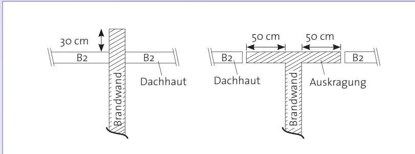
Abb. 2: Beispiele für die Ausbildung von Brandwänden im Dachbereich von Wohngebäuden und Gebäuden vergleichbarer Nutzung. Durch Brandwände soll die Weiterleitung eines Brandes auf den nächsten Brandabschnitt verhindert werden. (links: mindestens 30 cm über Dach geführte Brandwand, rechts: mit Auskragung ausgeführte Brandwand). Brennbare Baustoffe dürfen über die Brandwand bzw. die Auskragung nicht hinweggeführt werden (§ 30 [5] MBO). Die Kennzeichnung B2 entspricht der Baustoffklasse normalentflammbar nach DIN 4102. Insbesondere bei größeren Dachflächen bzw. Dachflächen über Grundstücksgrenzen ist zu prüfen, wo sich Brandwände befinden. Freistehende Einfamilienhäuser verfügen über keine Brandwände.
