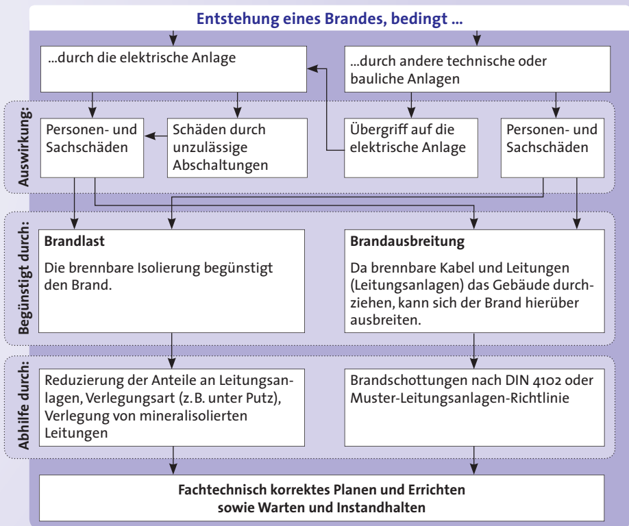
Abb. 1: Beteiligung einer elektrischen Anlage bei der Entstehung eines Brandes, bei der Brandentwicklung und bei der Brandweiterleitung, nach „Brandschutz in elektrischen Anlagen“, Herbert Schmolke, Hüthig & Pflaum
