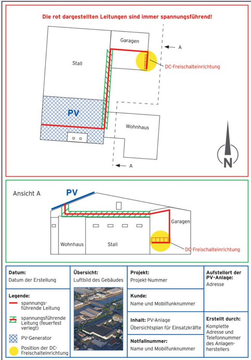
Abb. 8: Übersichtsplan für Einsatzkräfte (Muster)
