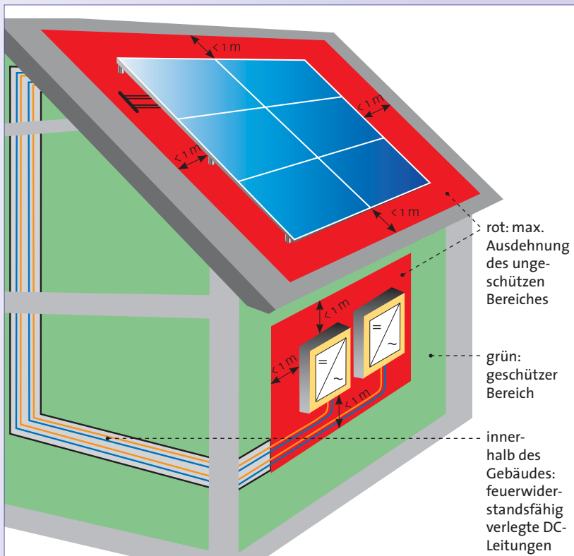
Abb. 5: Im Falle eines Isolationschadens (z. B. im Brandfall) können definierte Bereiche der PV-Anlage berührbare Spannungen führen. Diese definierten Bereiche sind im Abstand von maximal 1 m um den Wechselrichter bzw. 1 m um den PV-Generator zu realisieren. Darüber hinaus führende DC-Leitungen sollten entsprechend feuerwiderstandsfähig verlegt sein („geschützter Bereich“).
